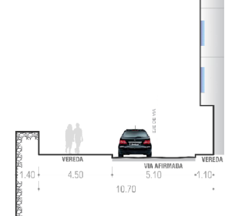
CORTE 24-23(D) VÍA PAVIMENTADA 10.70 ml
