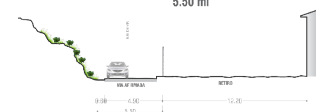
CORTE 19-19 CALLE 08 VÍA AFIRMADA 5.50 ml
