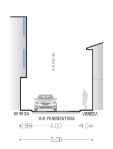
CORTE 17-17 CALLE 07 VÍA PAVIMENTADA 6.00 ml
